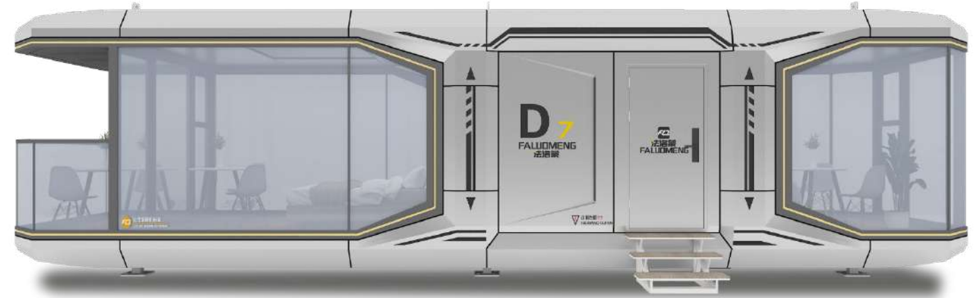
D7 长*宽*高 Length*Width*Height: 11.5*3.3*3.3 m 建筑面积 Building area: 37.95 m 2
