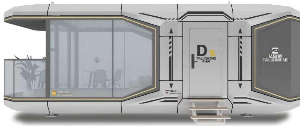
D5 长*宽*高 Length*Width*Height: 8.5*3.3*3.3m 建筑面积 Building area: 28.05 m 2
